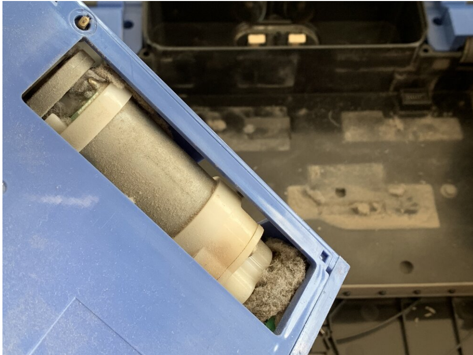
Let op hoeveel stof er rond de motor zit - het is als een warme winterjas...
