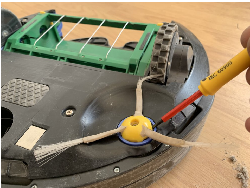
Wiebel de borstel los van zijn centrale as
