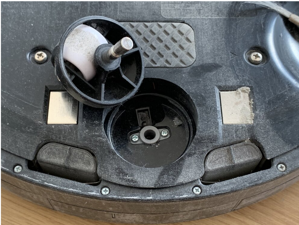
Verwijder stof van de sensor onder de wielbasis
