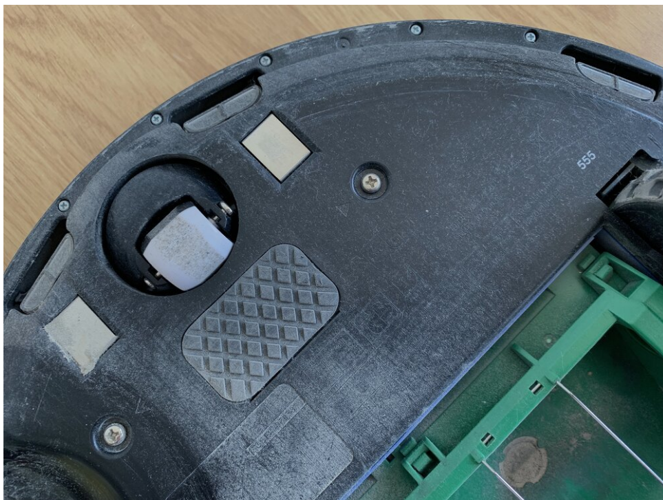
Maak "de ogen" van de Robot schoon, de sensorvensters bij de rand
