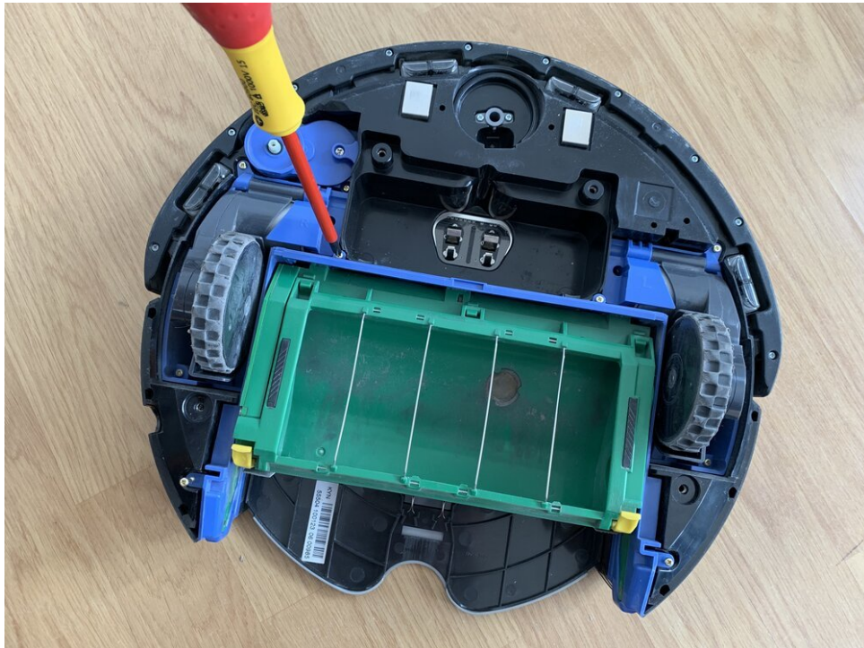
Verwijdering van de reinigingskop
